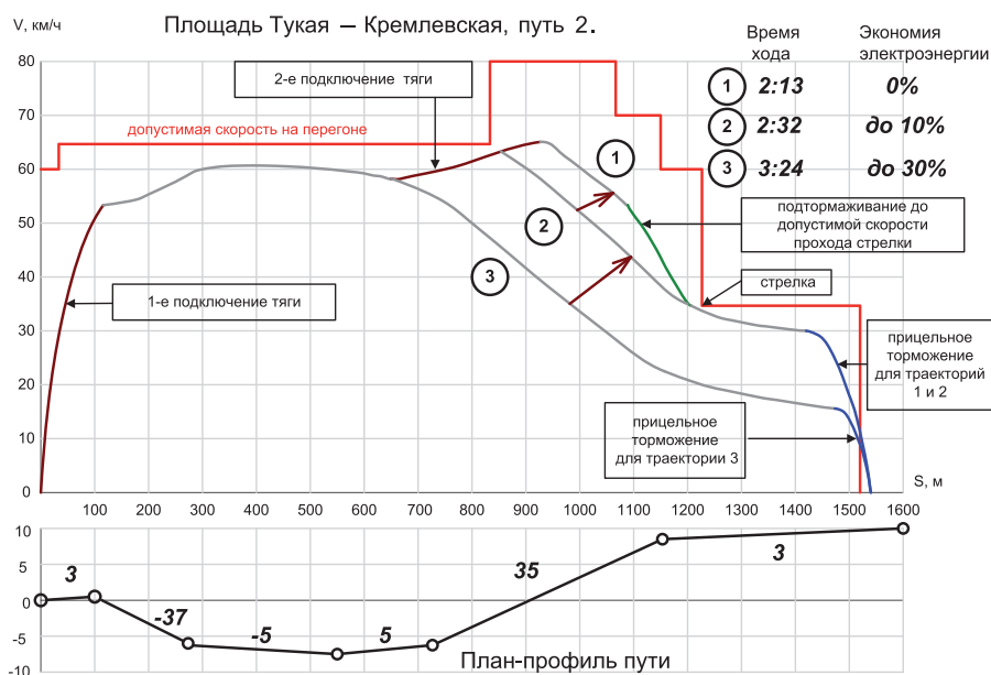
Рис. Графики прохождения перегона «Площадь Тукая» — «Кремлевская» по пути 2 для различных времен хода
